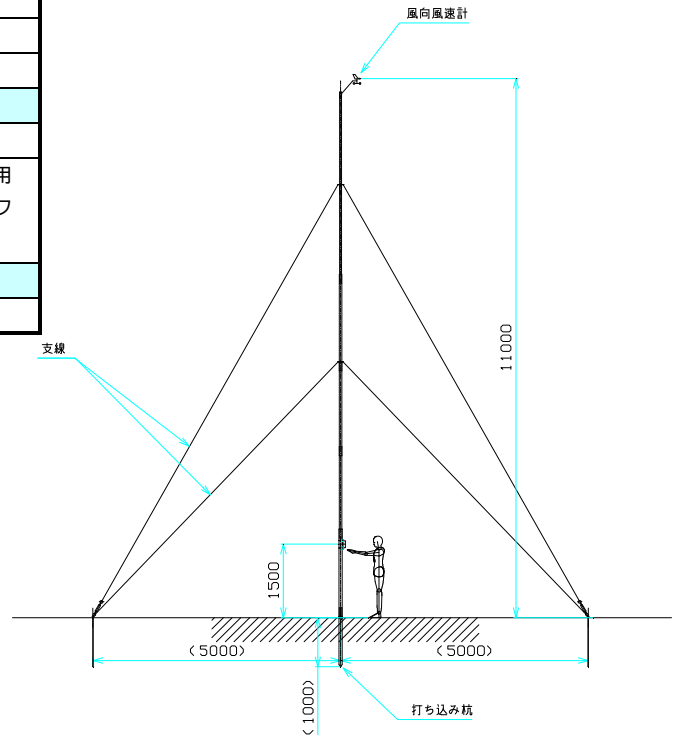
設置外観図
