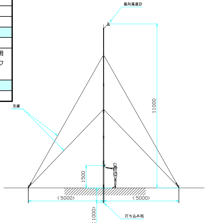
設置外観図
