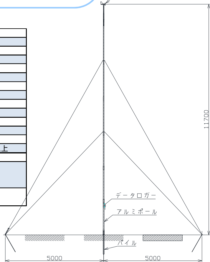
( 風向・風速計 )
